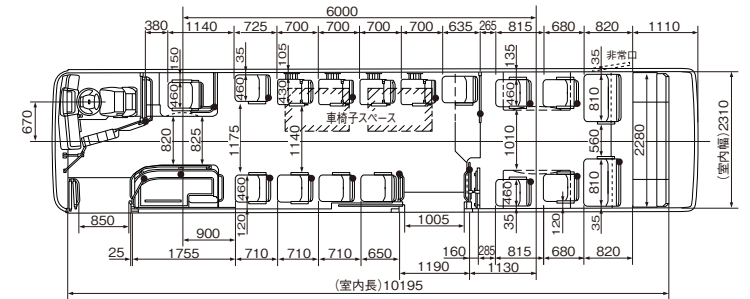
郊外II型 中乗 ホイールベース:6,000mm
