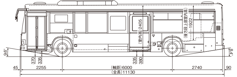
中乗 ホイールベース:6,000mm
