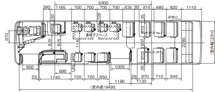
ラッシュ型 前乗 ホイールベース:5,300mm
