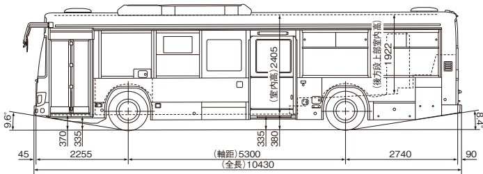
中乗 ホイールベース:5,300mm
