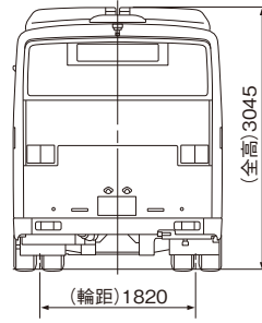
前乗 ホイールベース:6,000mm
