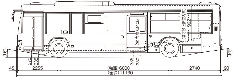
中乗 ホイールベース:6,000mm
