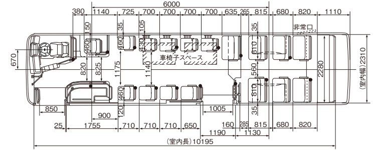
ラッシュ型 中乗 ホイールベース:6,000mm
