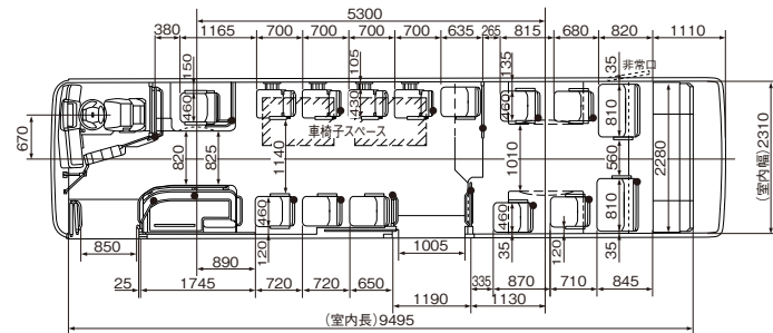
郊外I型 中乗 ホイールベース:5,300mm
