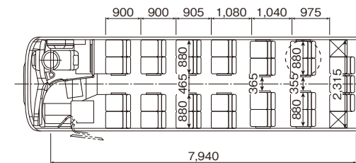
■HD-9【貸切】 後部2列サロン席 7列 スイング扉 カタログ番号【10】
