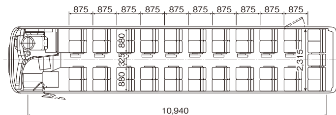
■HD【貸切】 前向席 11列 スイング扉 カタログ番号【1】
