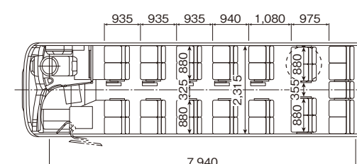
■HD-9【貸切】 後部2列サロン席 7列 スイング扉 カタログ番号【10】
