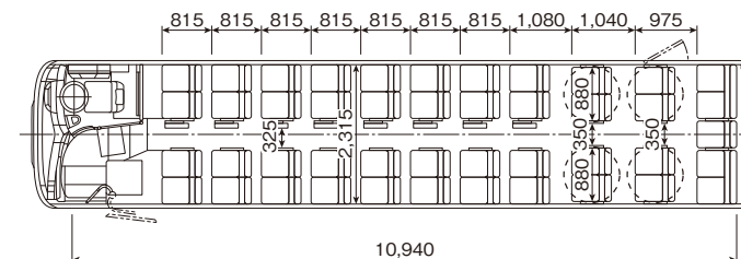
■HD-VP【貸切】 後部2列サロン席 11列 スイング扉 カタログ番号【14】
