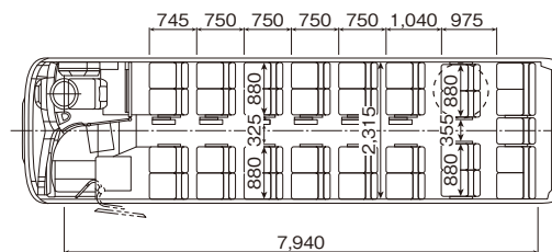
■HD-9【貸切】 後部スライド2列サロン席 8列 スイング扉 カタログ番号【11】
