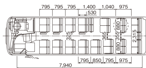
■HD-9【貸切】 後部スライド2列サロン席 8列 スイング扉 カタログ番号【11】
