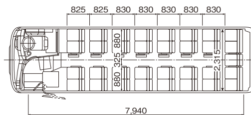
■HD-9【貸切】 後部1列サロン席 8列 スイング扉 カタログ番号【9】
