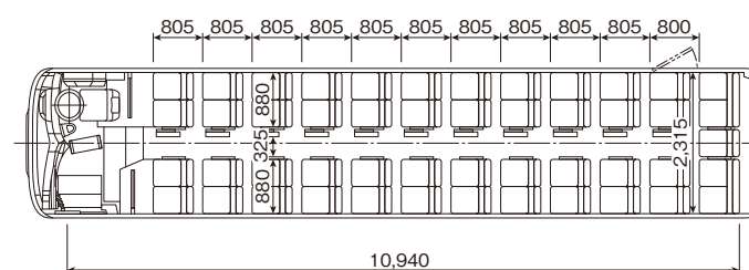
■HD-VP【高速路線】 トイレ無し 12列 折扉 カタログ番号【27】
